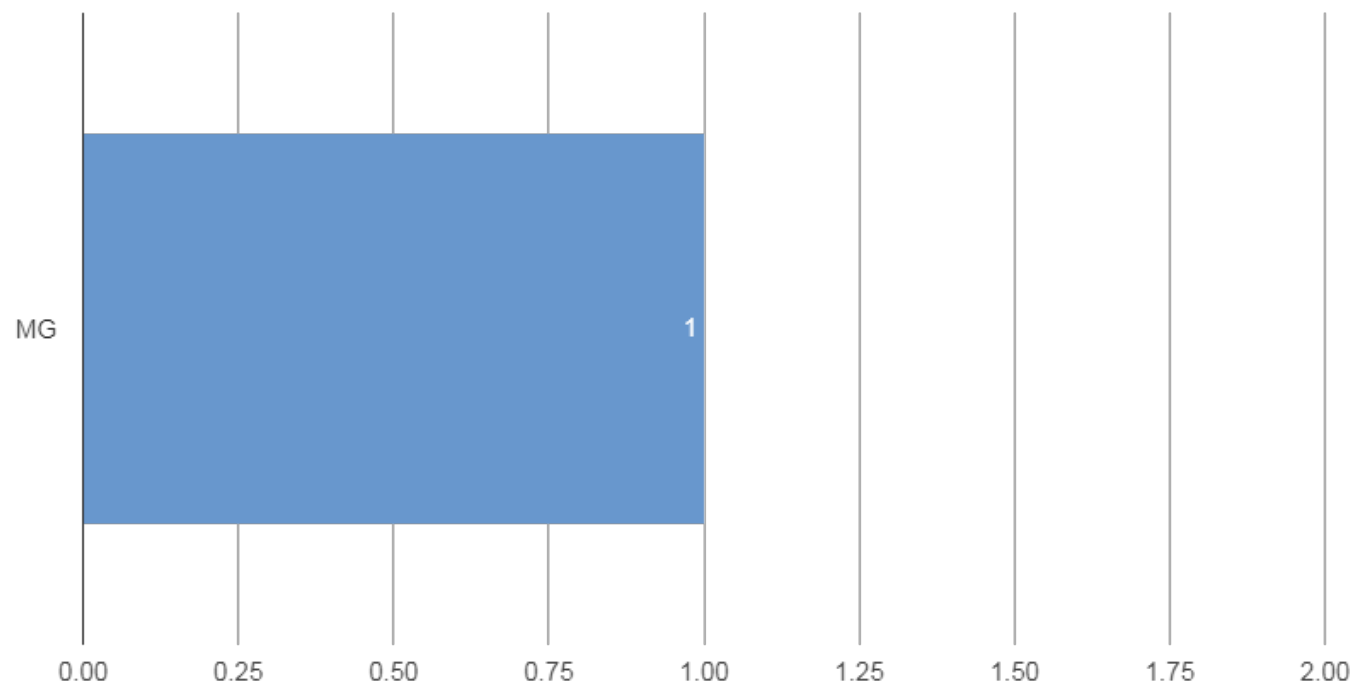
Estado (5 maiores)
